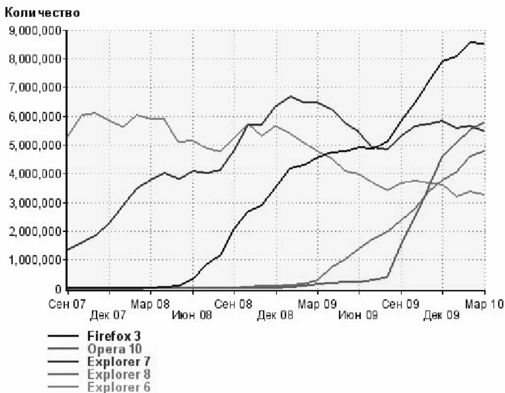
Рис. 1.2. Статистика использования браузеров в Рунете (http://www.liveinternet.ru/)
